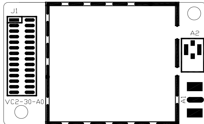
图 1.引脚位置图
