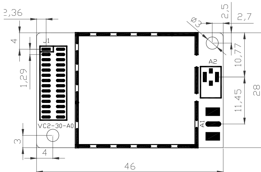
图 2.产品尺寸图
